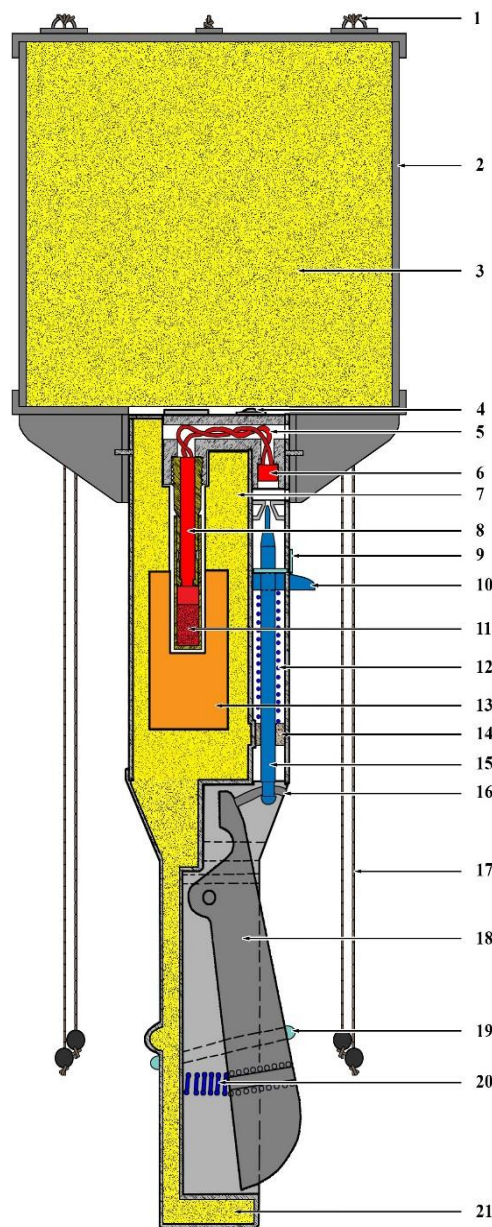
Ruční granát Rdultovskij vz. 1914, s přídatnou hlavicí k ničení drátěných překážek:
